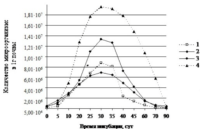
Рис. 1 - Изменение численности экологических групп микроорганизмов почвы при орошении жидкой фракцией БН дозой по азоту 200 мг/дм 3 : 1 – микроскопические грибы (среда Чапека); 2 – олигокарбофилы (ГА); 3 – микроорганизмы круговорота азота (КАА); 4 – гетеротрофы (МПА)
